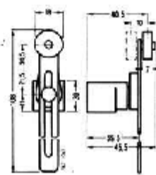
Kol uzunluğu ayarlı makara tahriki
