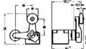
Çift makaralı tahriki
