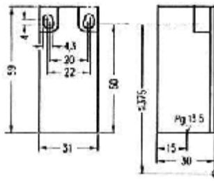
3SE3 200
